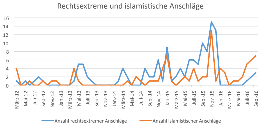
Abbildung 1: Analyse der GDT-Daten für die USA, Australien, Deutschland, Großbritannien und Frankreich
